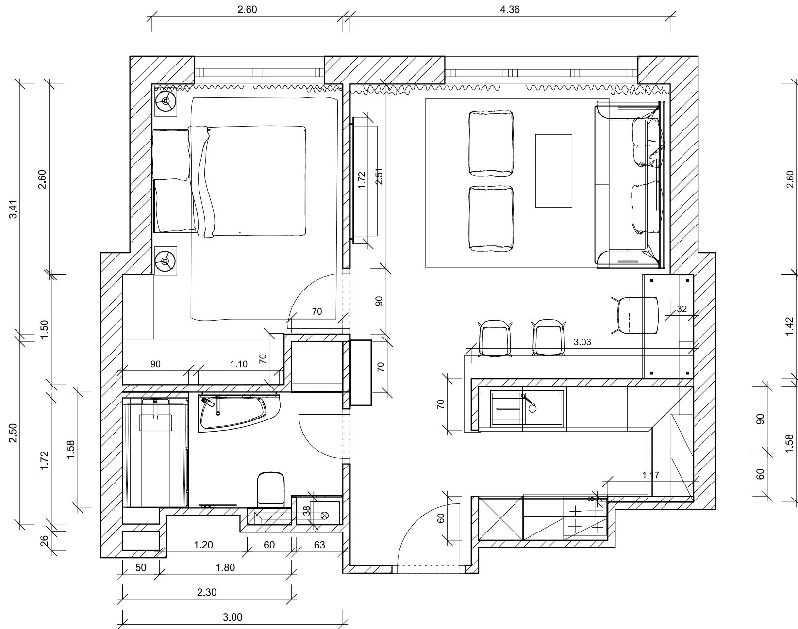
86230 Méretezett berendezési terv 1:50
